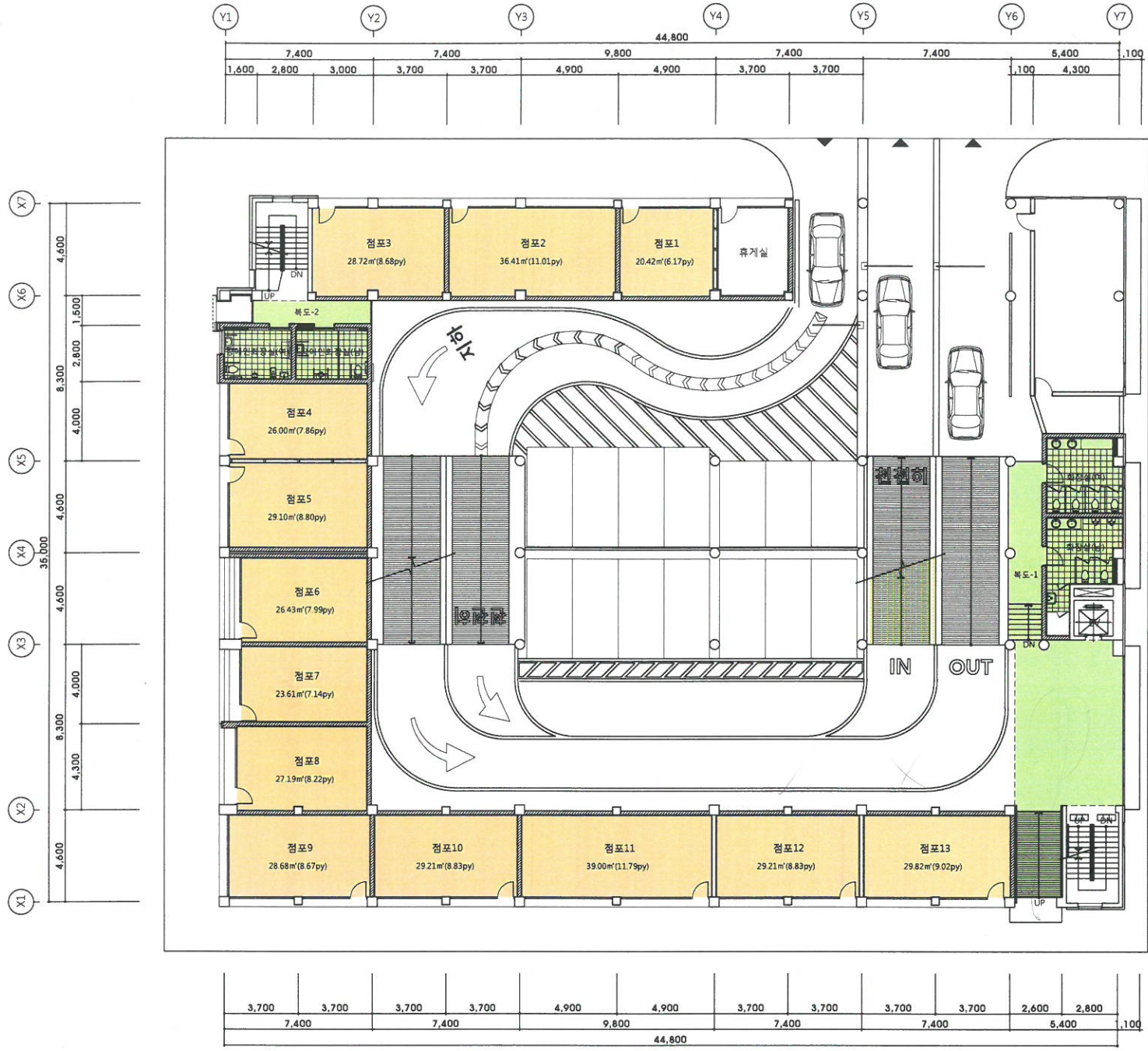
1 지상1층 평면도(신설) SCALE : 1/200
